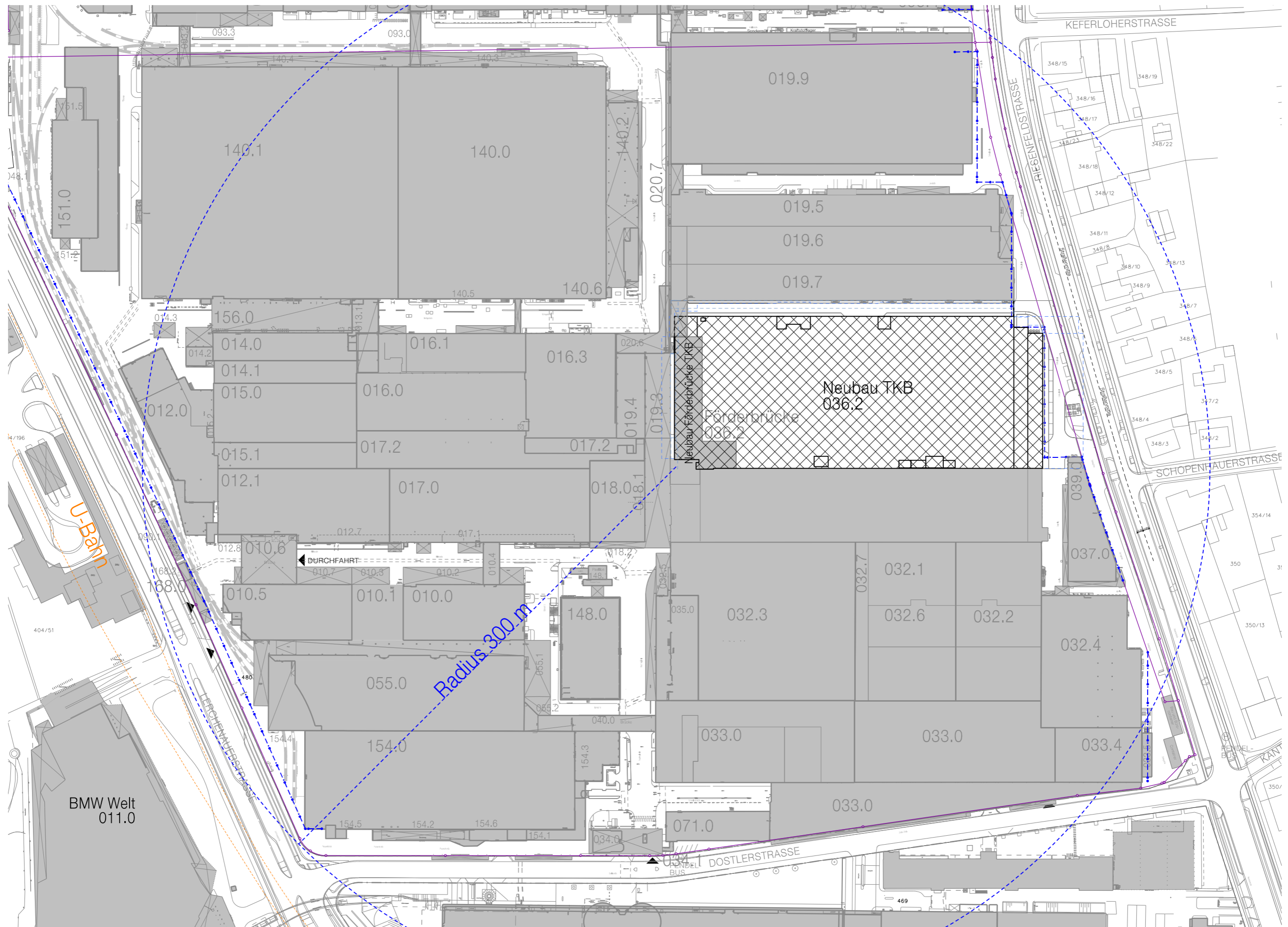
Auszug Lageplan BMW München, Werk 01.10, Neubau Gebäude 36.2, Karosseriebau TKB
