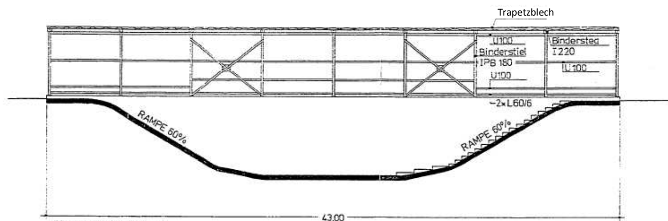
LÄNGSSCHNITT A-A longitudinal section A-A
