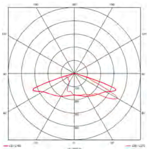
Beispiel-Lichtverteilung T-M
