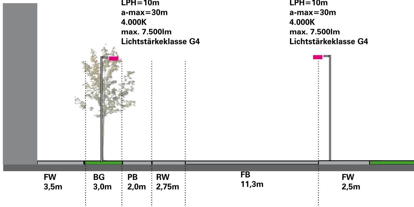
Beispiel-Lichtverteilung T-M
