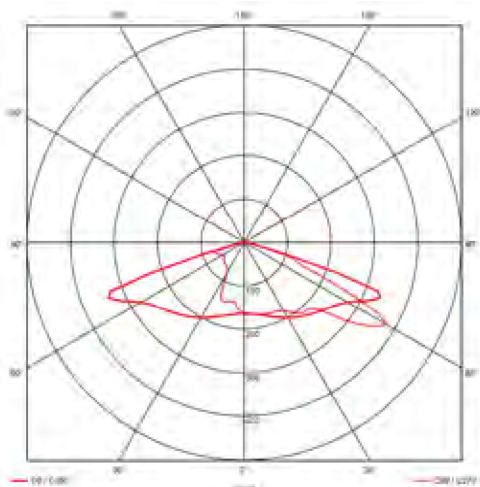
Beispiel-Lichtverteilung T-M
