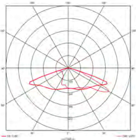
Beispiel-Lichtverteilung T-M
