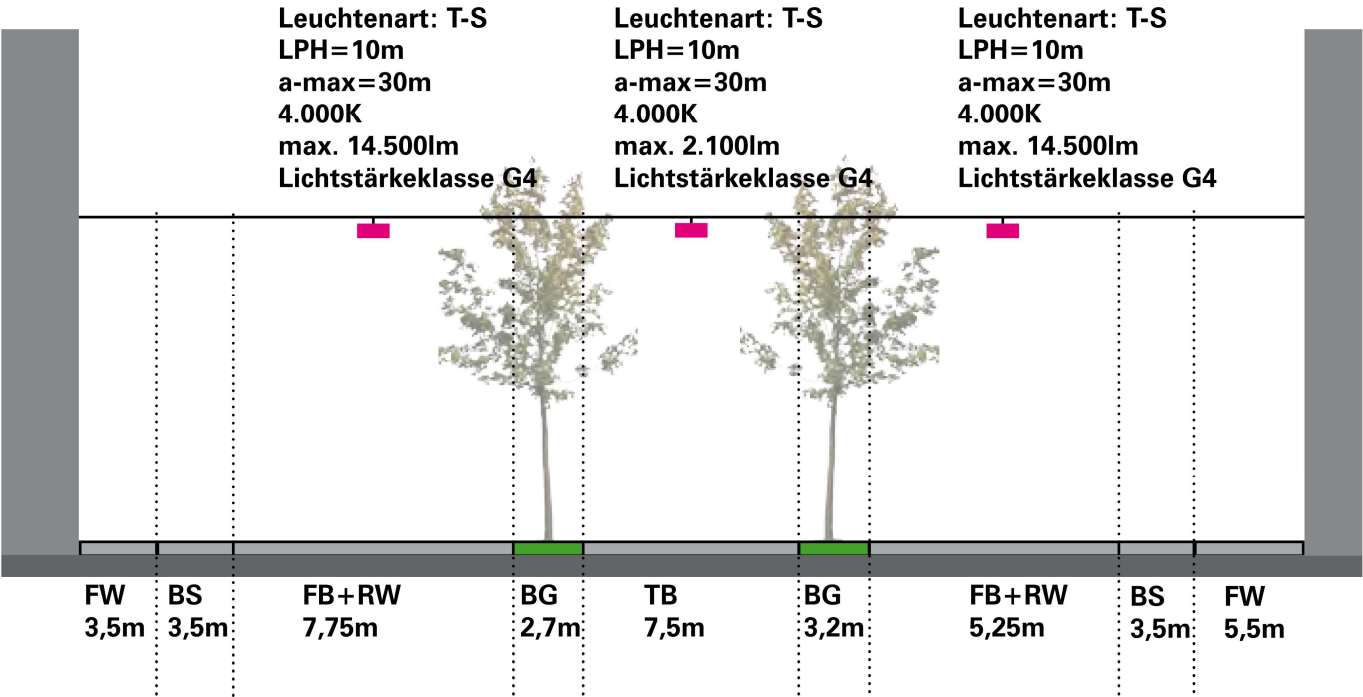
Beispiel-Lichtverteilung T-S
