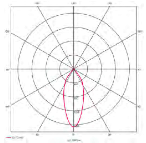
Beispiel-Lichtverteilung G-M
