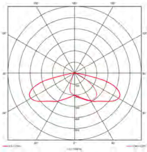
Beispiel-Lichtverteilung T-M
