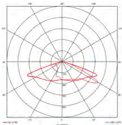
Beispiel-Lichtverteilung T-M
