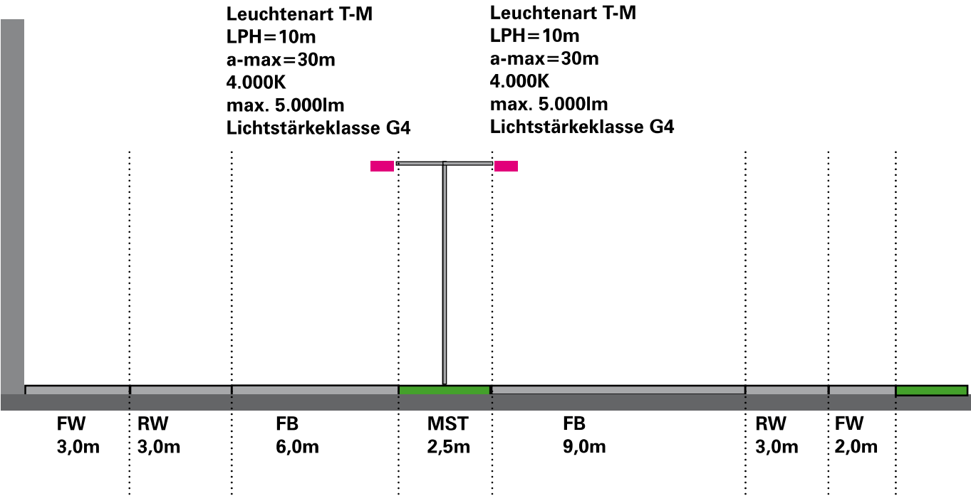
Beispiel-Lichtverteilung T-M
