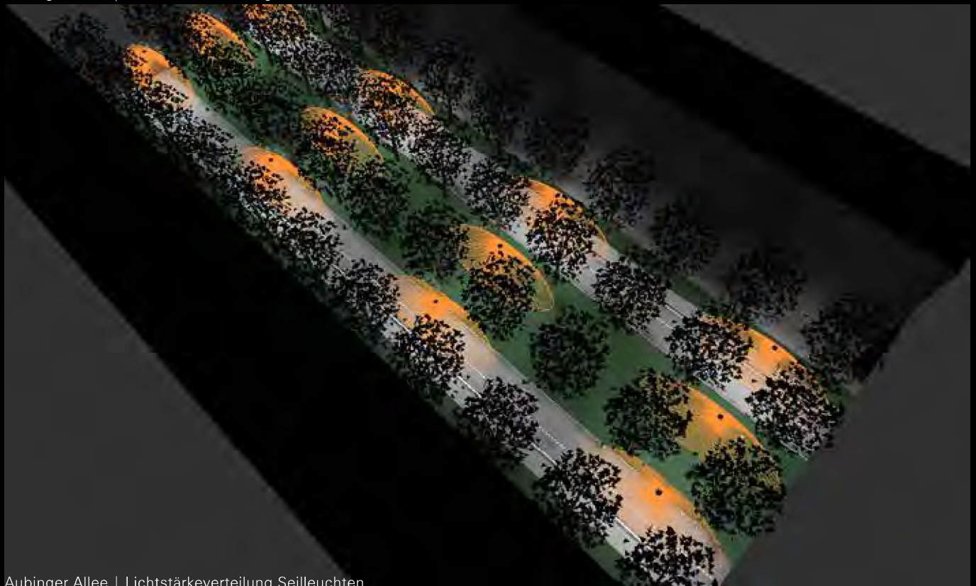
Aubinger Allee | Lichtstärkeverteilung Seilleuchten
