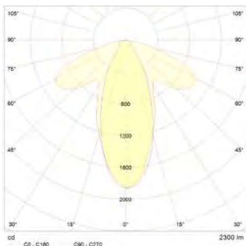
Beispiel-Lichtverteilung G-M
