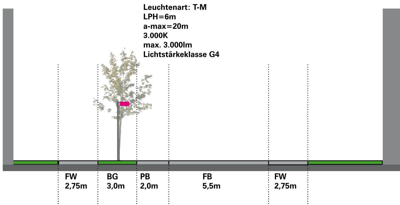
Beispiel-Lichtverteilung T-M
