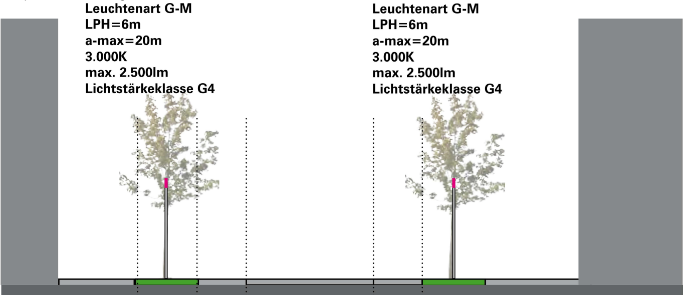
Beispiel-Lichtverteilung G-M
