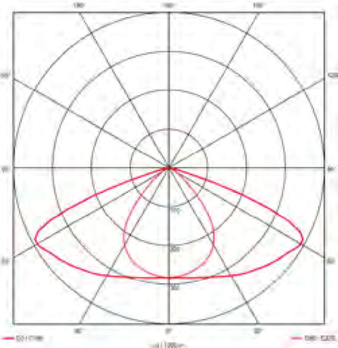
Beispiel-Lichtverteilung T-S
