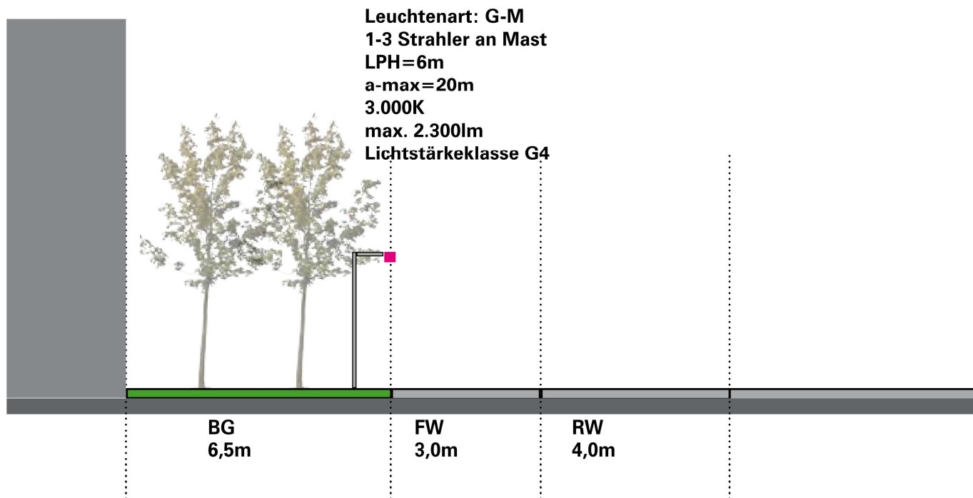
Beispiel-Lichtverteilung G-M
