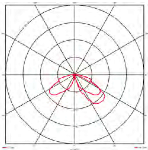
Beispiel-Lichtverteilung G-M
