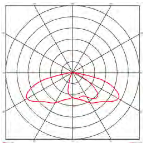
Beispiel-Lichtverteilung T-M
