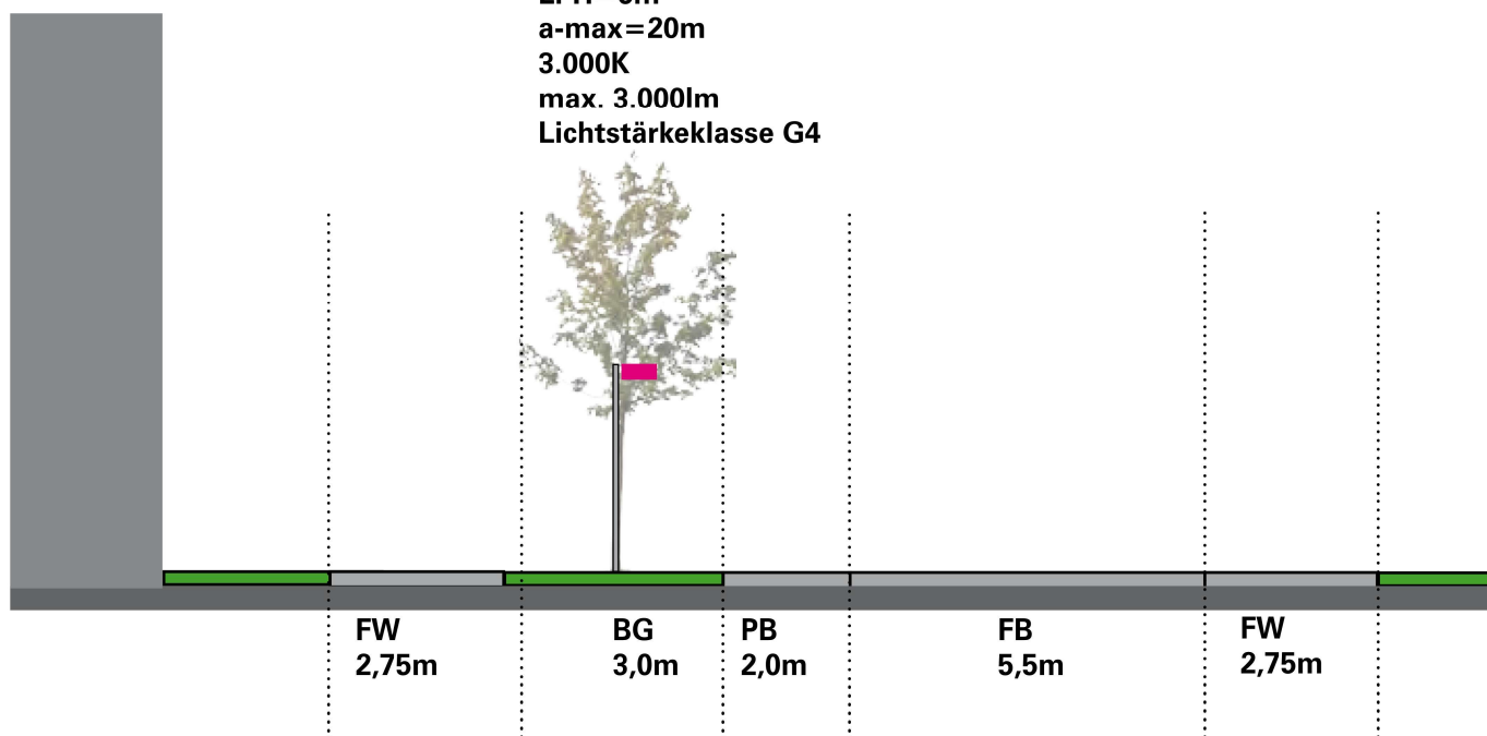
Beispiel-Lichtverteilung T-M
