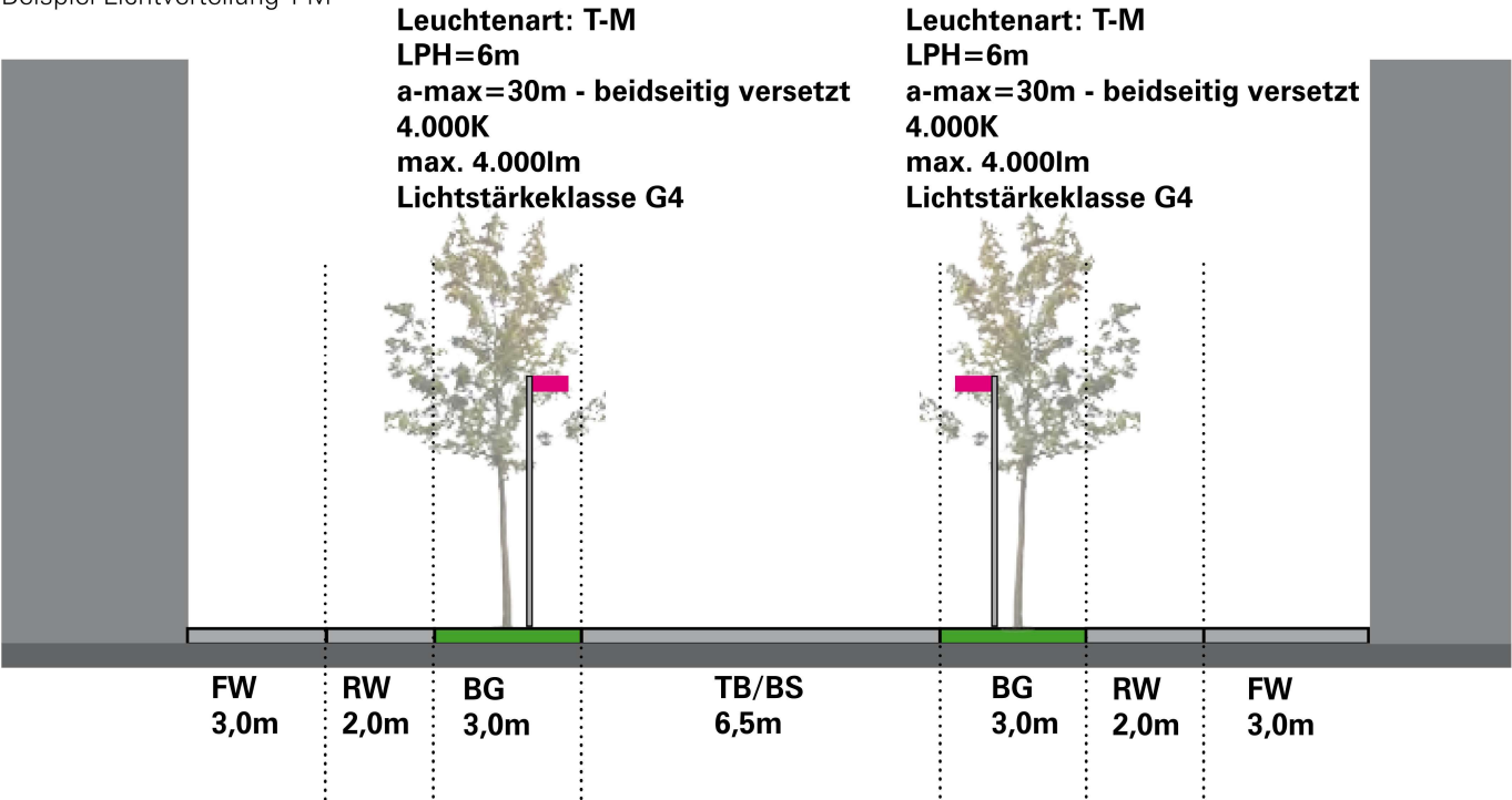
Beispiel-Lichtverteilung T-M
