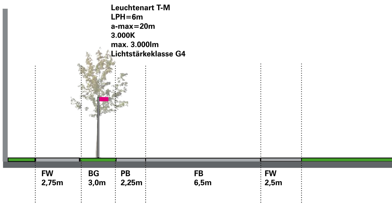
Beispiel-Lichtverteilung T-M
