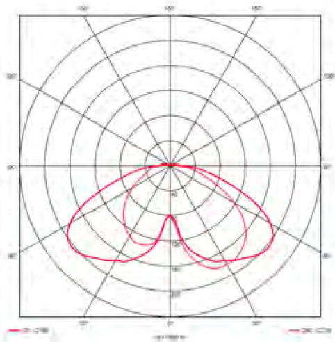
Beispiel-Lichtverteilung G-M
