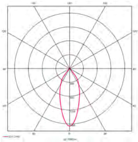
Beispiel-Lichtverteilung G-M
