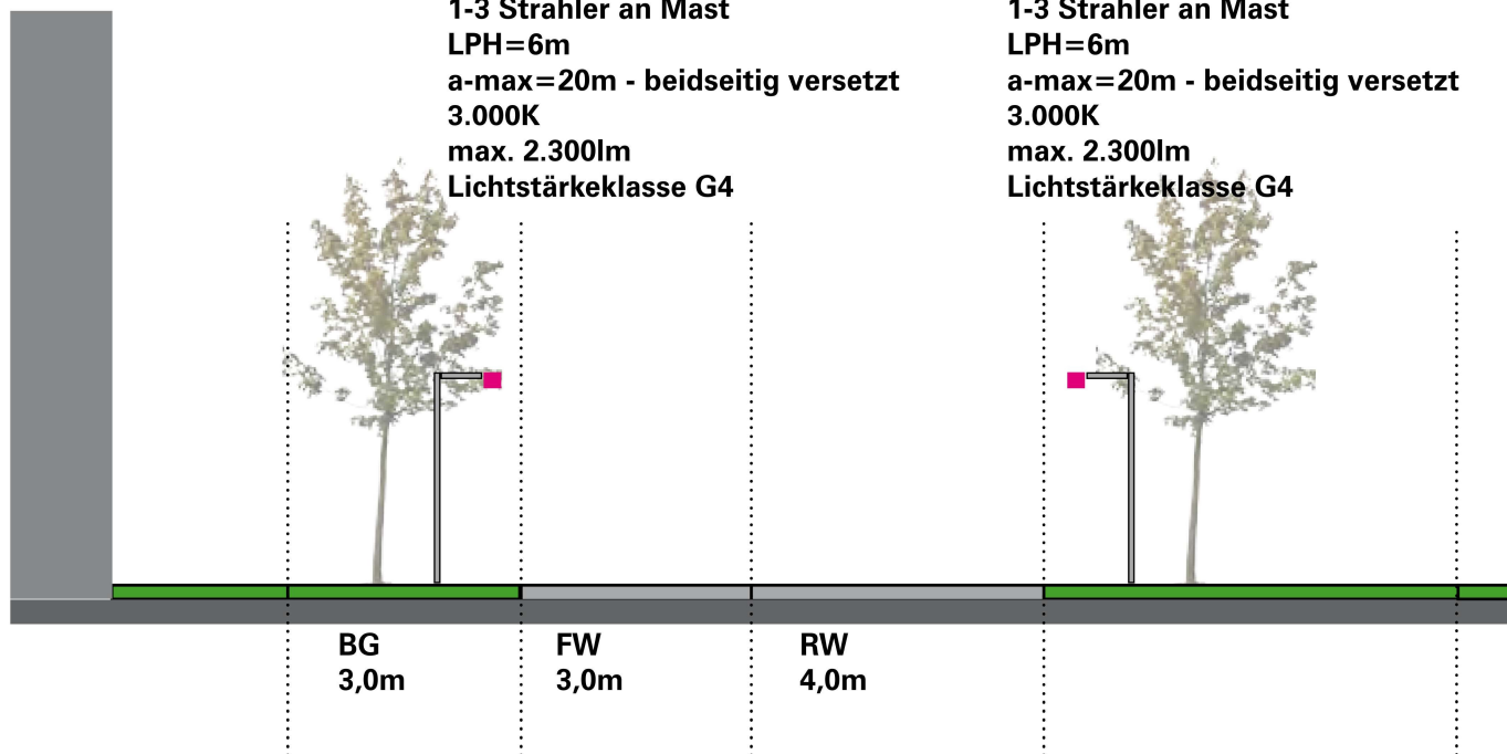
Beispiel-Lichtverteilung G-M
