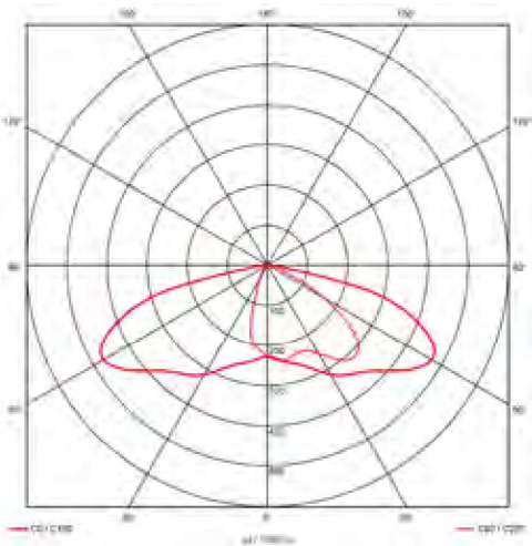
Beispiel-Lichtverteilung T-M
