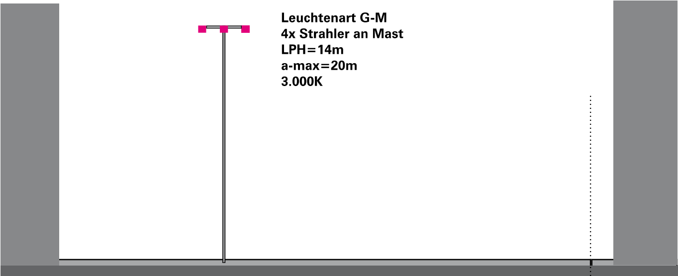
Beispiel-Lichtverteilung G-M Strahler
