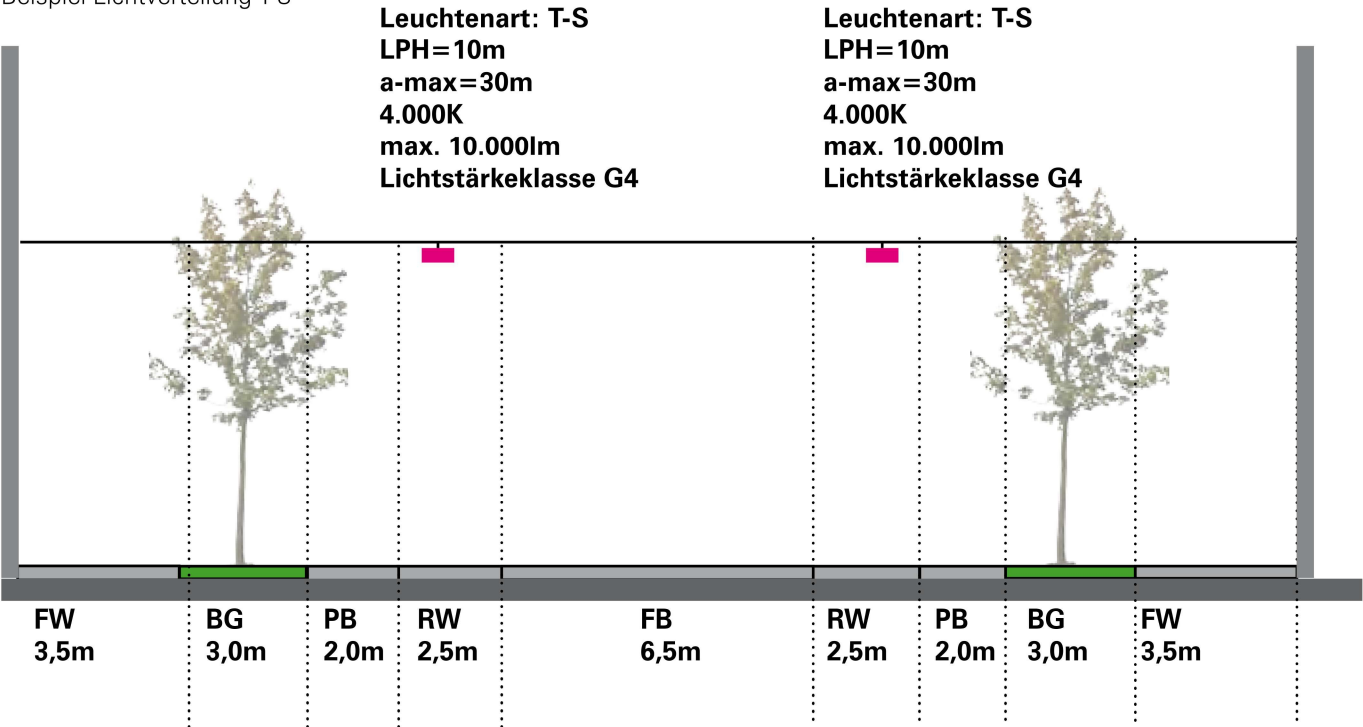
Beispiel-Lichtverteilung T-S
