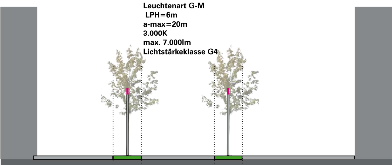
Beispiel-Lichtverteilung G-M
