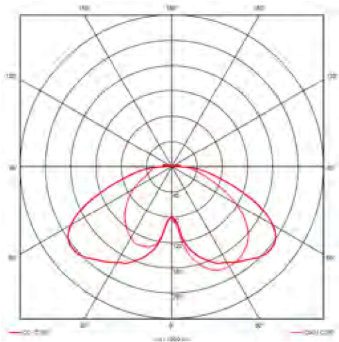
Beispiel-Lichtverteilung G-M
