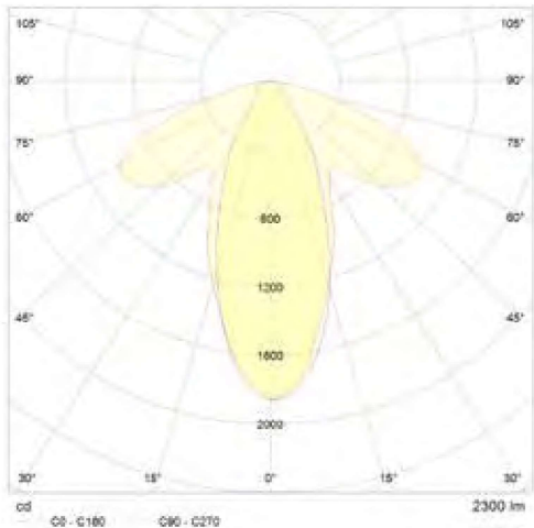
Beispiel-Lichtverteilung G-M Strahler
