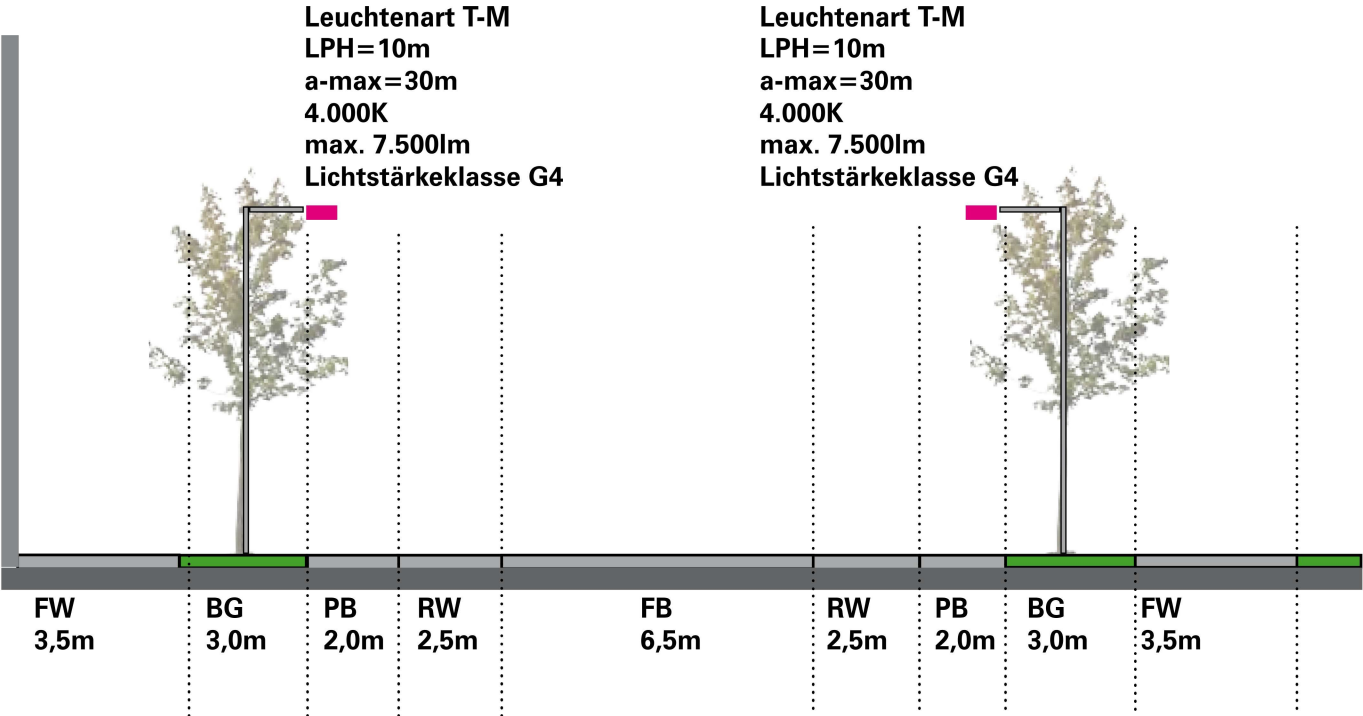
Beispiel-Lichtverteilung T-M
