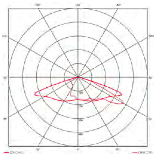
Beispiel-Lichtverteilung T-M
