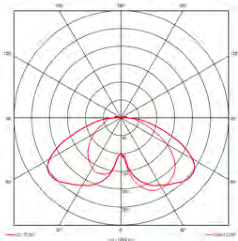
Beispiel-Lichtverteilung G-M
