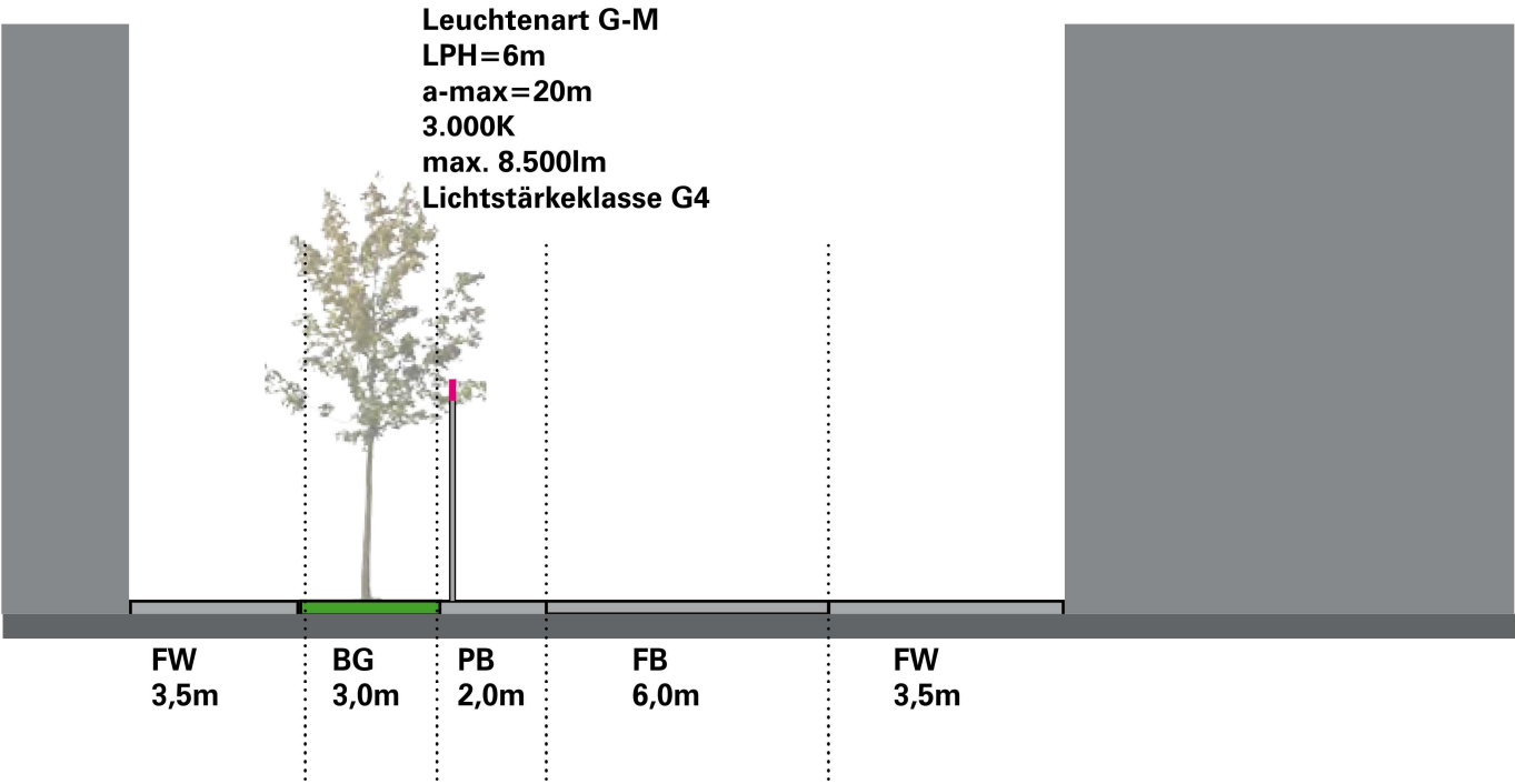
Beispiel-Lichtverteilung G-M
