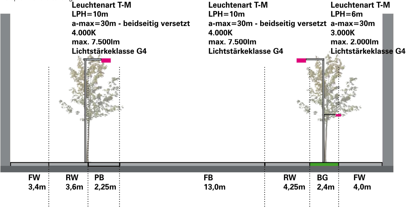
Beispiel-Lichtverteilung T-M
